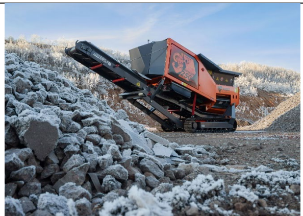
Der kompakte Zweiwellenzerkleinerer im Special Dunmow-Design (Foto: ARJES)
